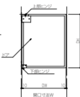
立面図
