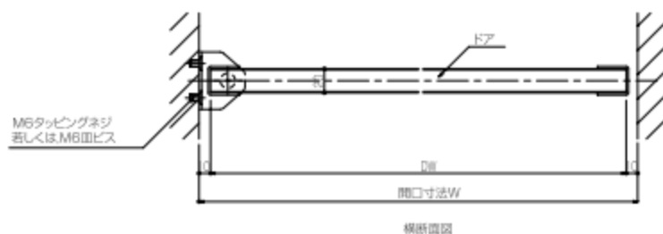
横断面図
