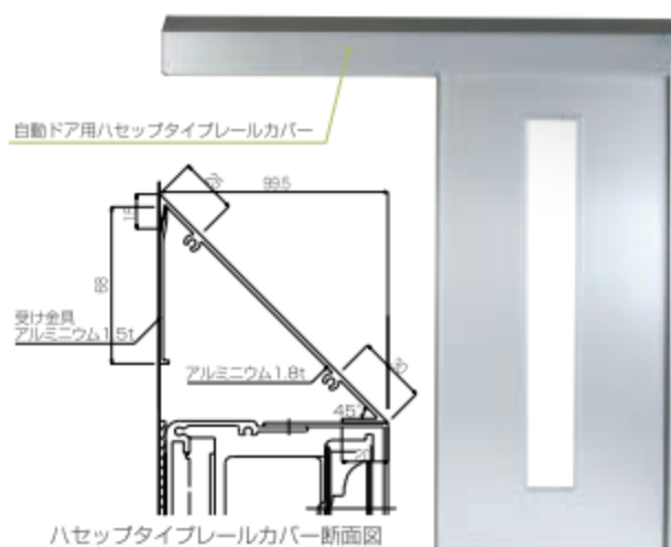
写真は自動ドア表面材:アルミニウム、ドア厚 t=30\text{mm} 、自動ドア用ハセップタイプレールカバー仕様
