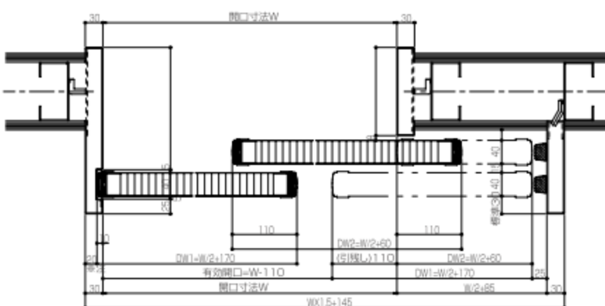
2連式外付右引横断面図
