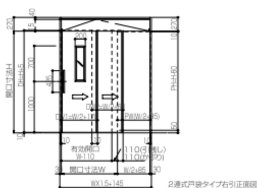
2連式戸袋タイプ右引正面図
