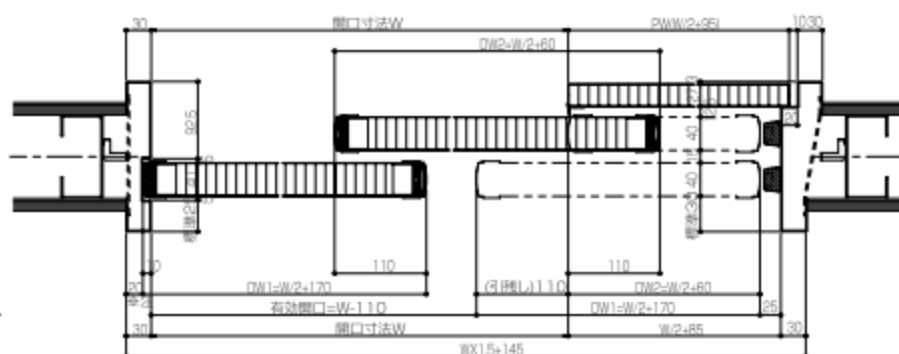
2連式戸袋タイプ右引横断面図
