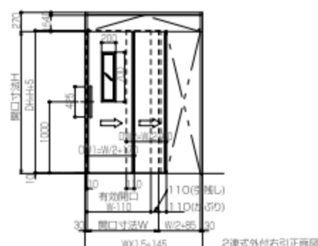
2連式外付右引正面図
