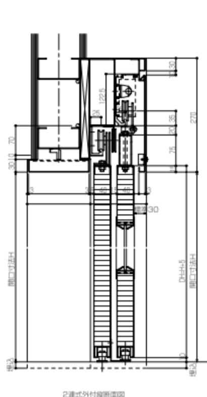
2連式外付タイプ正面図
