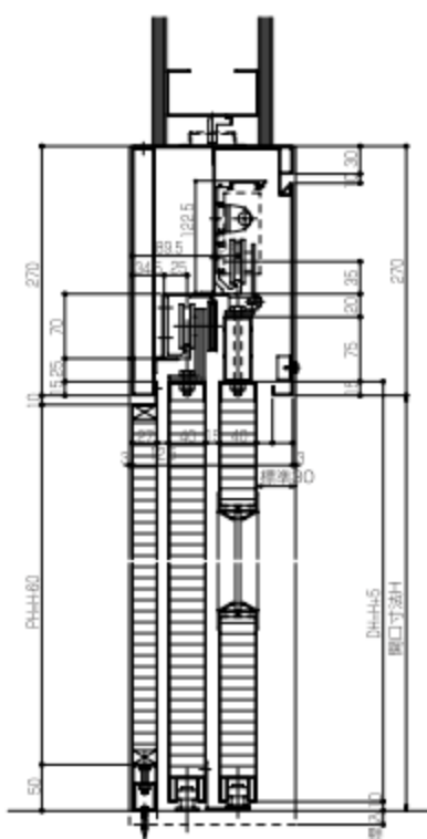
2連式戸袋タイプ正面図
