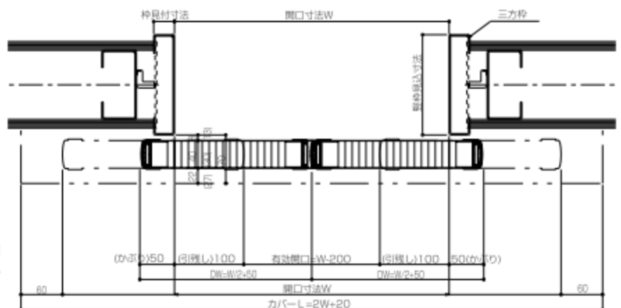
両引標準横断面図
