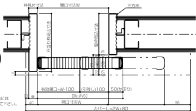
右引標準横断面図
