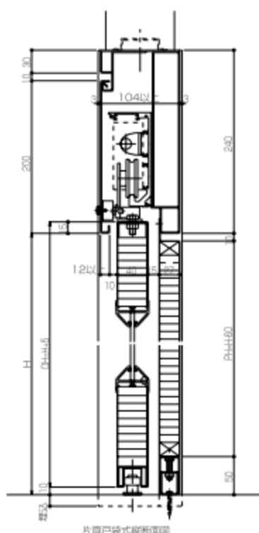
片面戸袋式スライドドア図面
