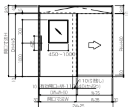
片面戸袋式右引正面図
