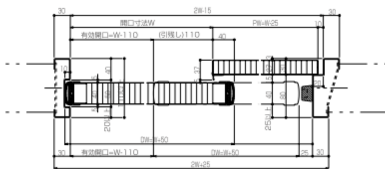
片面戸袋式右引横断面図
