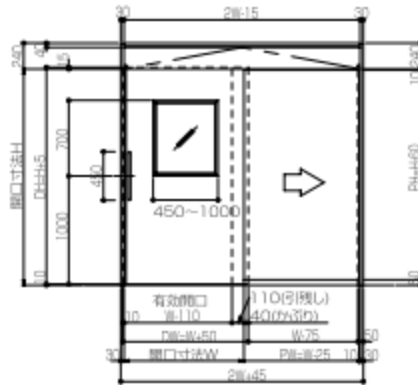
片面戸袋片面壁式右引正面図
