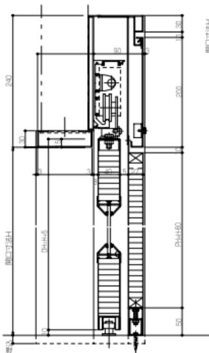
片面戸袋片面壁式扉断面図
