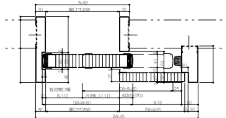
片面戸袋片面壁式右引横断面図
