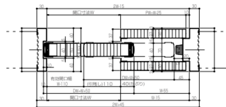
両面戸袋式横断面図
