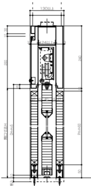
両面戸袋式扉断面図
