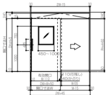
両面戸袋式正面図
